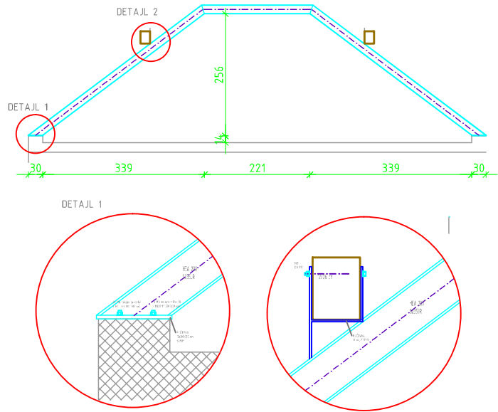
JEKLEN OKVIR NAD GALERIJO – 2 kos M 1:50
